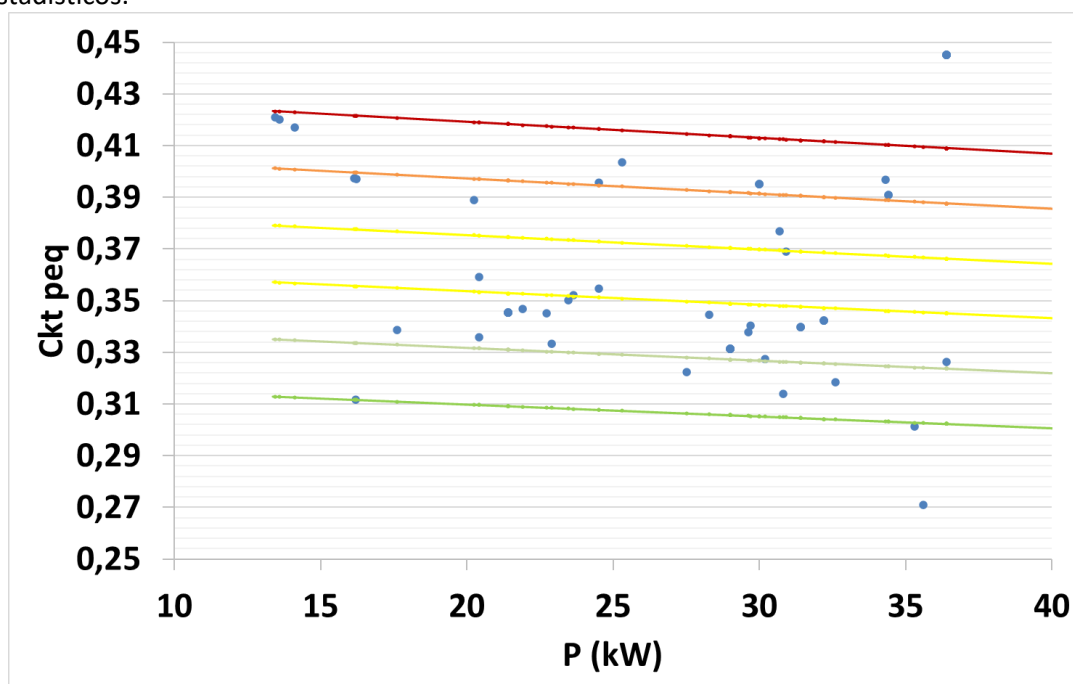
Fig. 3 Estado actual de las zonas de clasificación energética de tractores de menos de 2500 kg.
