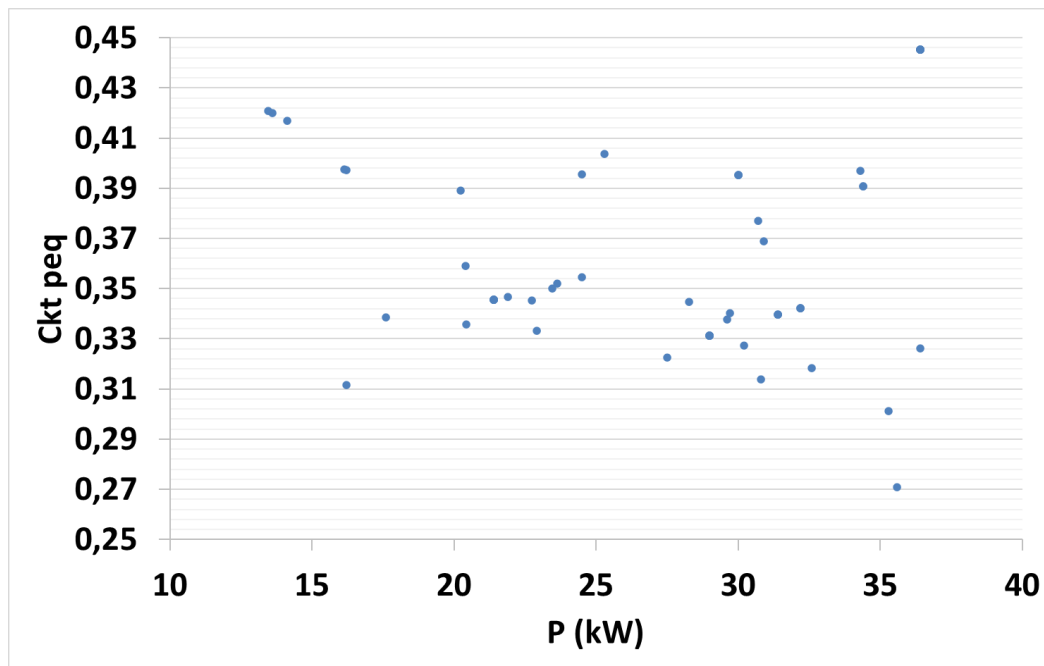
Fig. 2 Diagrama con nube de puntos de los modelos de tractor de menos de 2500 kg clasificados.
