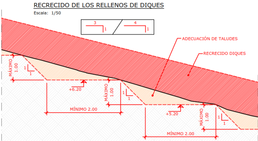
Figura 53. Abancalamiento previo a ejecutar en los diques a recrecer.
