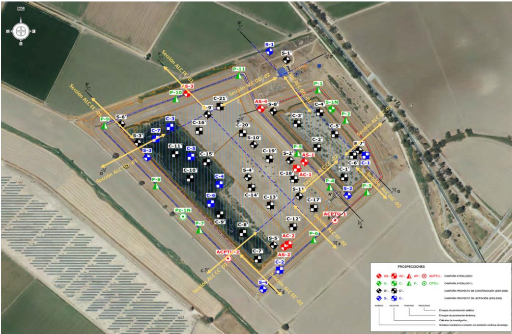
Figura 57. Imagen de la Balsa de Alcantarilla con indicación de los trabajos realizados y secciones de cálculo.
