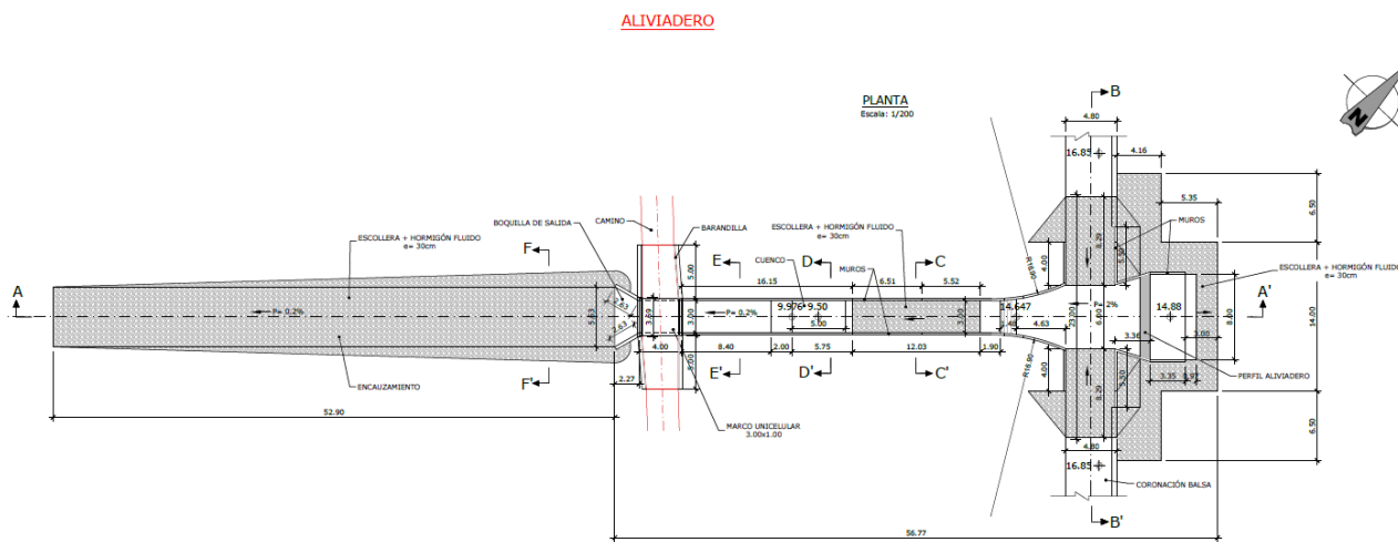
Figura 45: Aliviadero balsa de regulación. Planta. S, Alcantarillas
