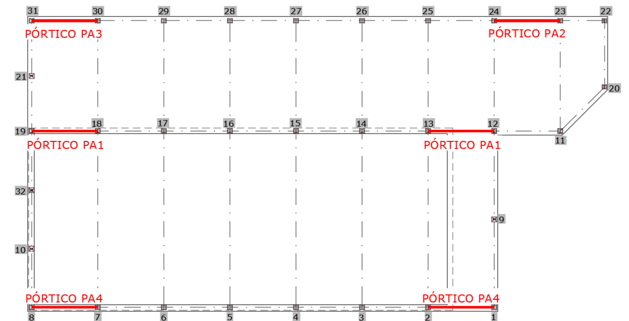
Ilustración 1: Pórticos de la estructura metálica que no cuentan con las cruces de San Andrés. Elementos a reponer.
