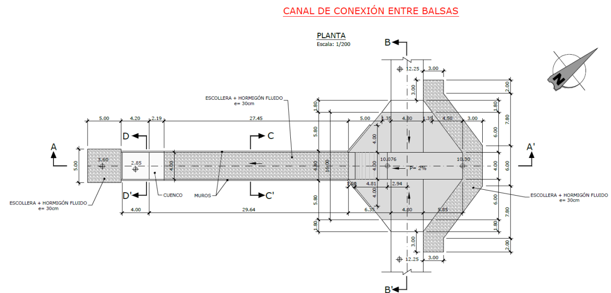
Figura 35: Canal de interconexión entre balsas. S. Belmonte
