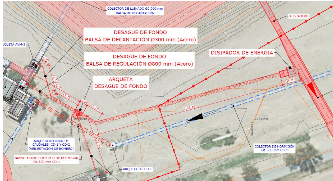
Figura 36: Layout de los desagües de los nuevos desagües de fondo de la balsa de decantación y regulación
