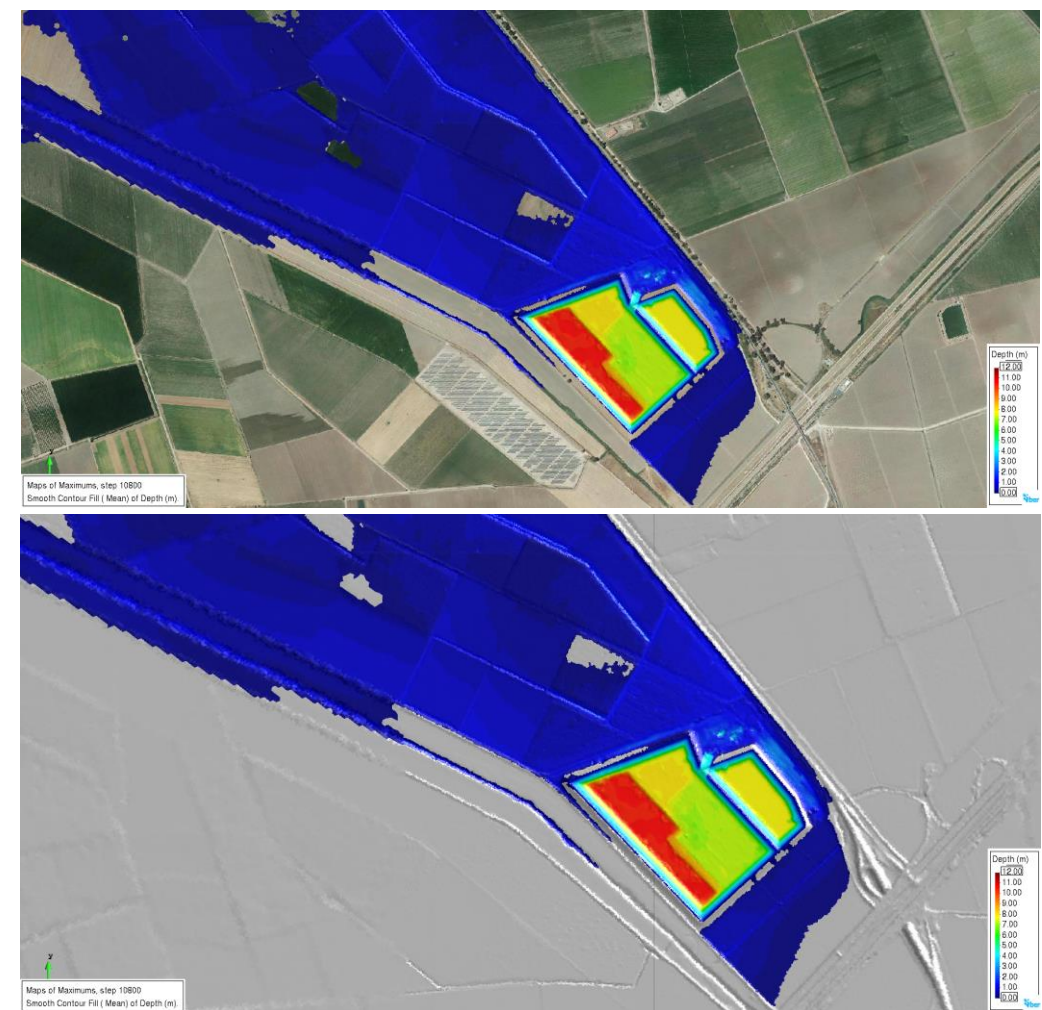
Figura 59. Máximos calados alcanzados en la rotura 1
