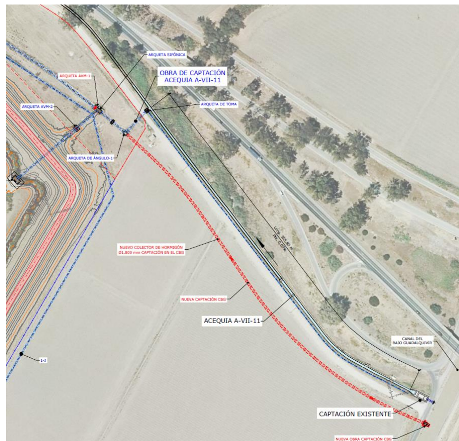
Figura 39: Planta de situación de las obras de captación del sector Alcantarillas. Existente en acequia A-VII-11 y nueva captación paralela
