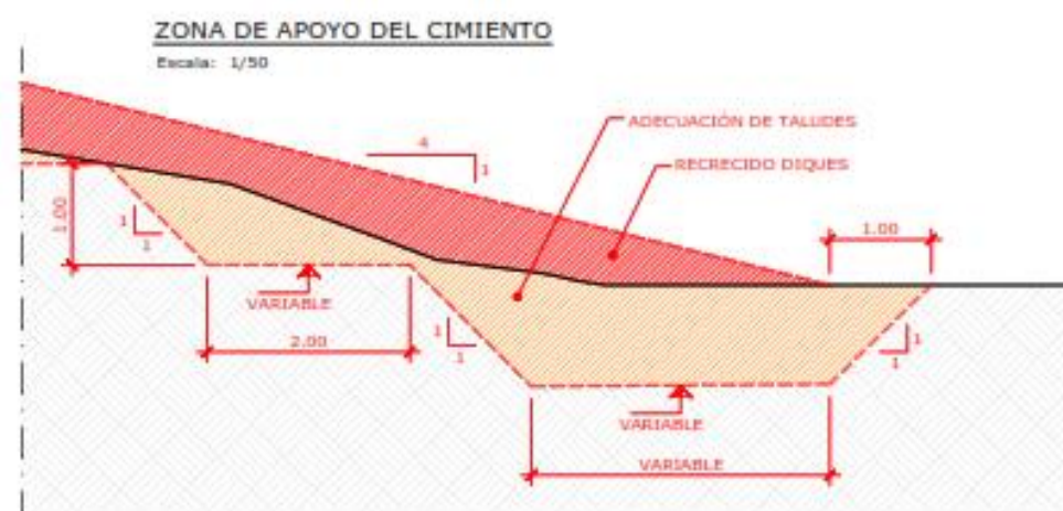
Figura 54. Detalle del saneo en el pie de apoyo del recrecido a ejecutar de manera previa.
