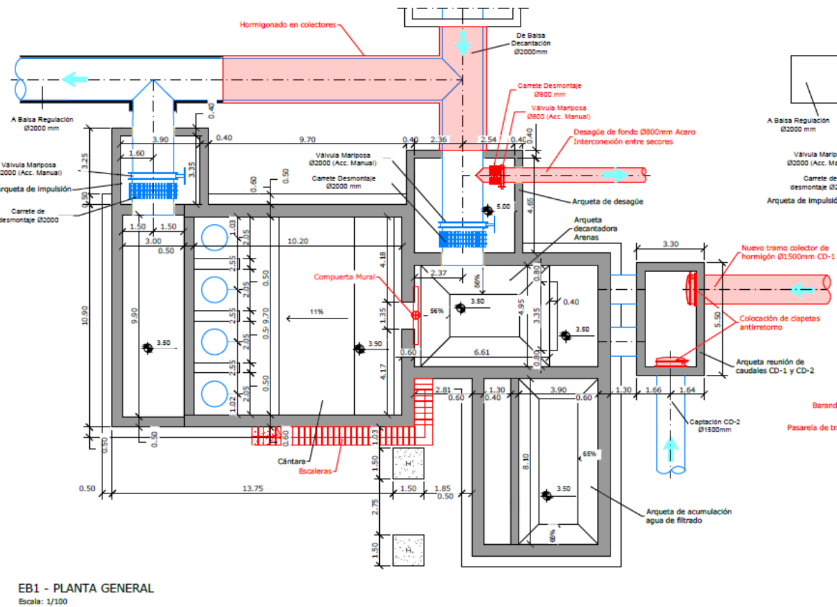
Figura 28. Planta estación de bombeo de llenado
