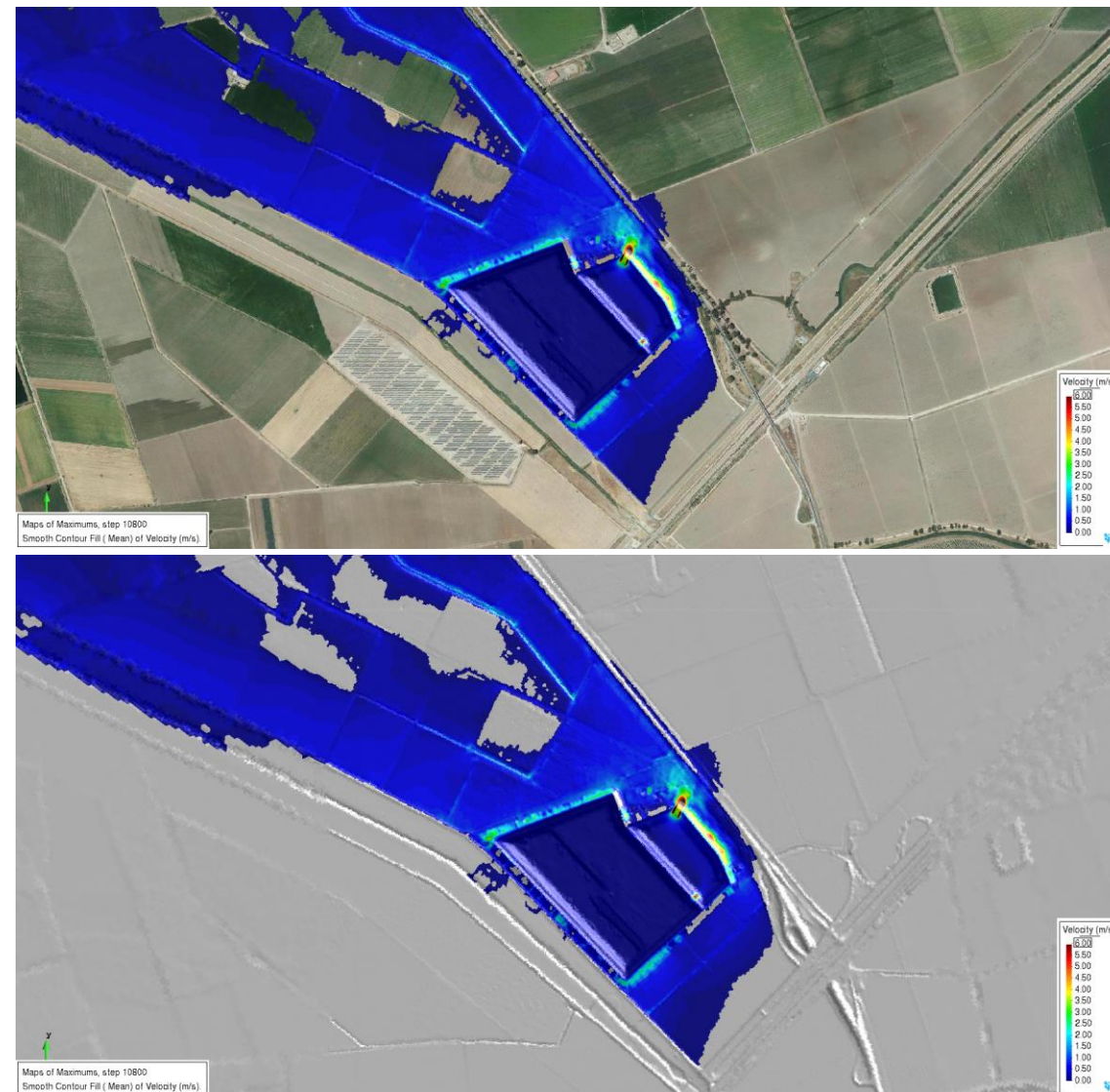
Figura 61. Máximas velocidades alcanzadas en la rotura 4 en estado actual
