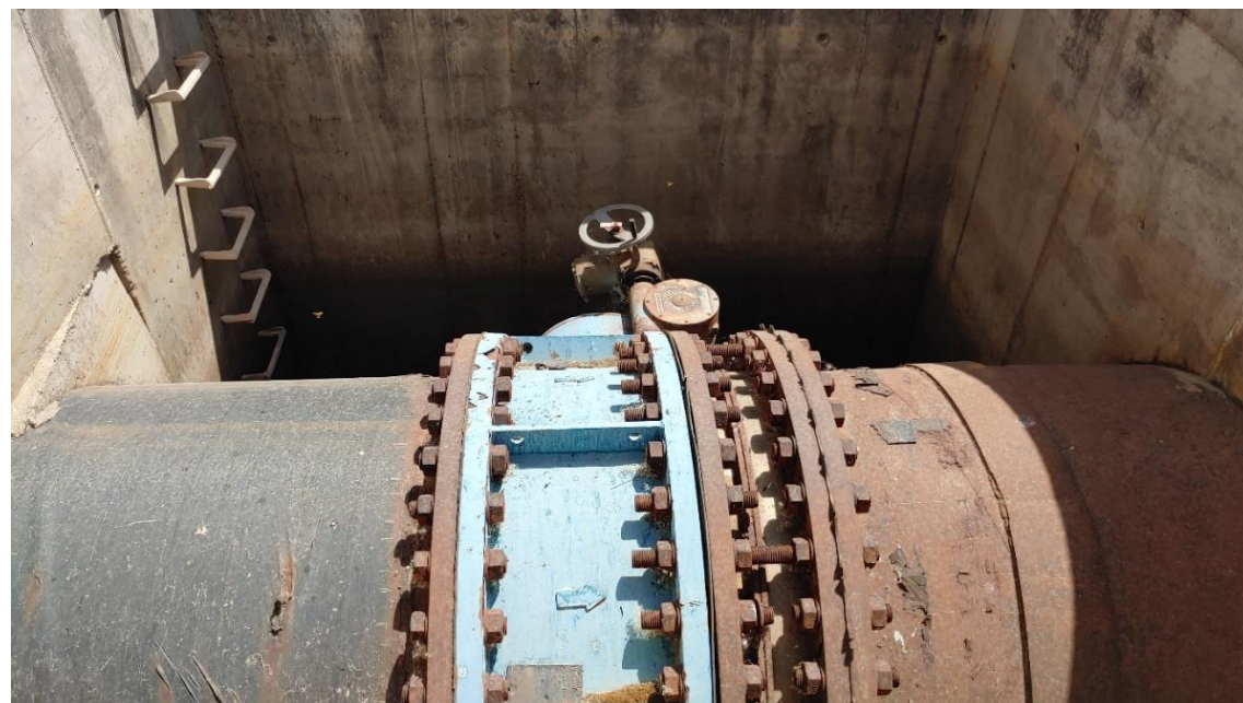
Figura 12. Estado actual de la Arqueta V.M. 4 (2)
