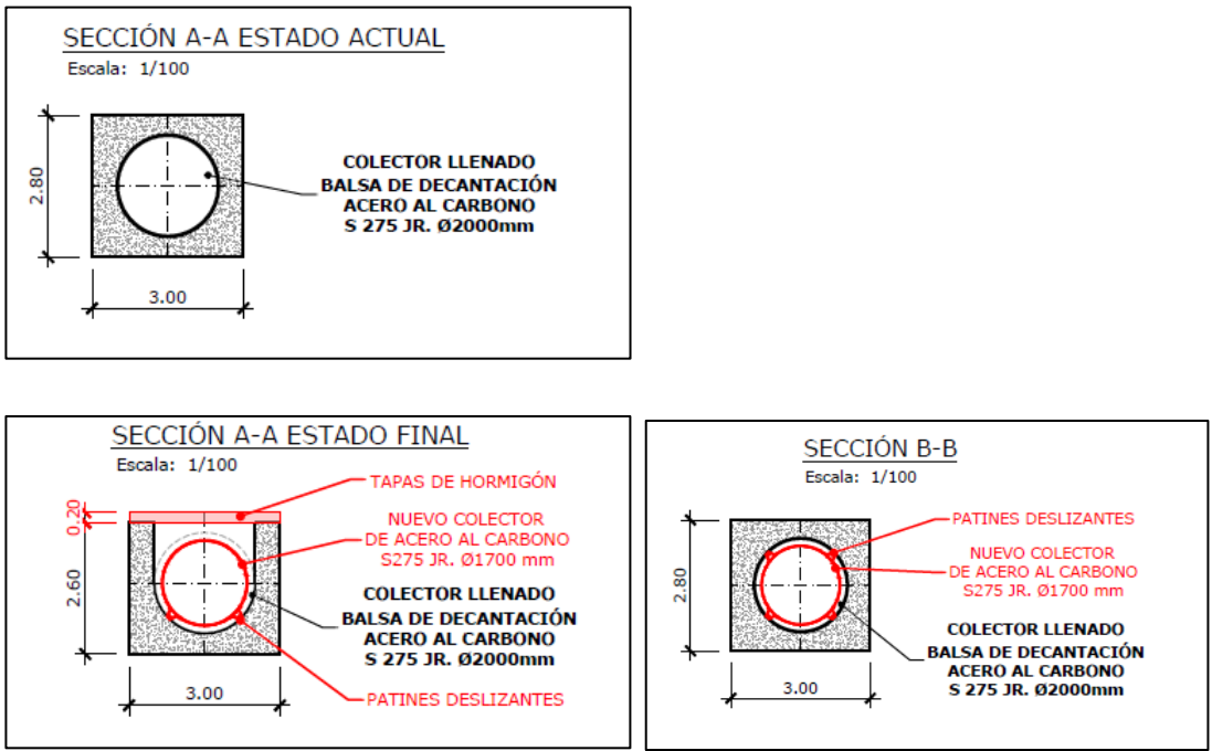
Ilustración 3: Secciones tipo del colector de fondo . Estado actual y estado proyectado, mediante nueva camisa de acero interior
