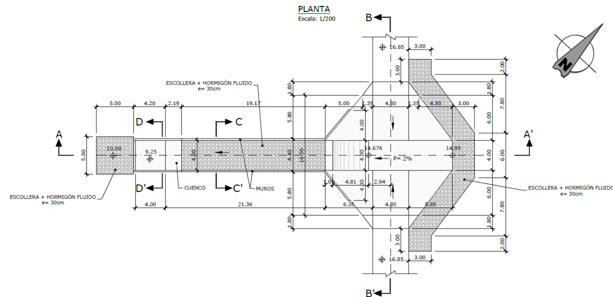
Figura 47: Canal de interconexión entre balsas. S. Alcantarillas
