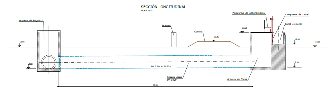
Figura 40. Obra de captación en acequia A-VII-11
