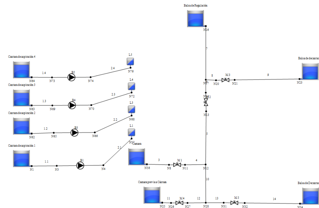
Figura 64. Representación esquemática del sistema en estudio.
