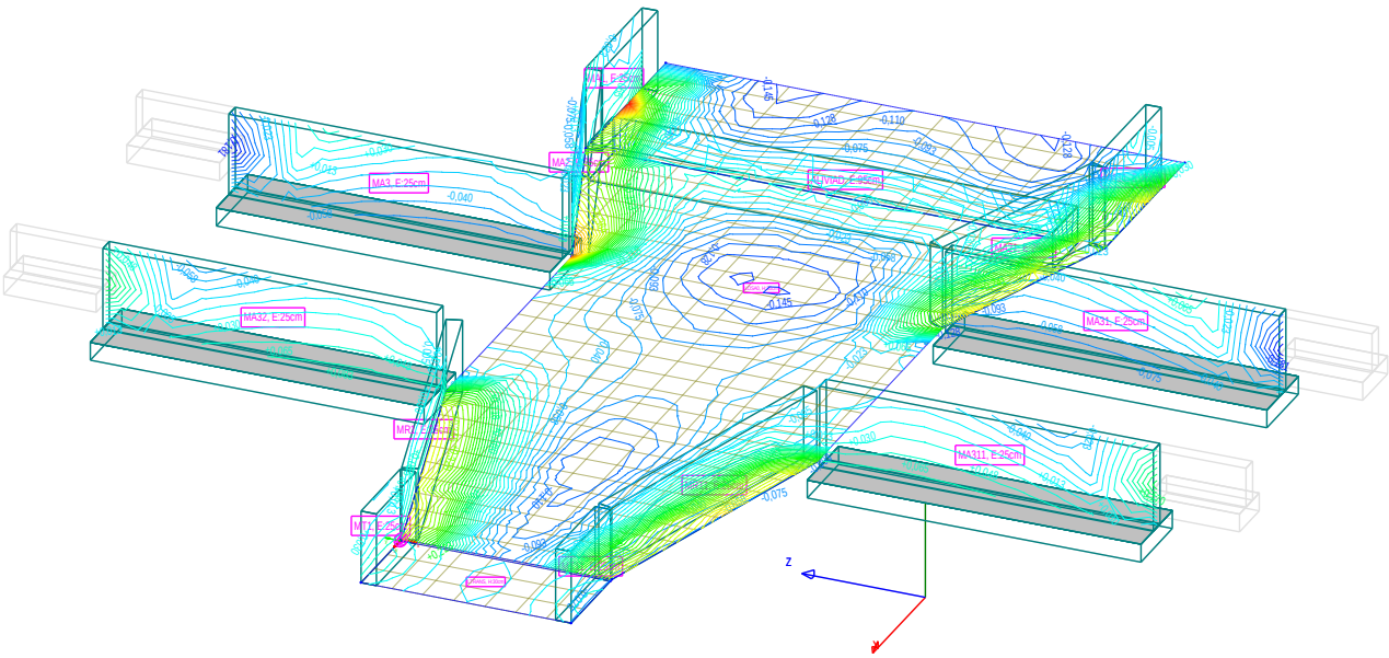
Ilustración 5: Modelo de Calculo estructural del aliviadero de la Balsa Belmonte
