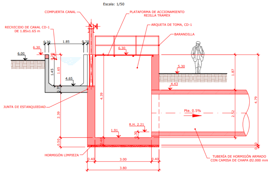
Figura 24. Obra de captación en canal de derivación CD-1
