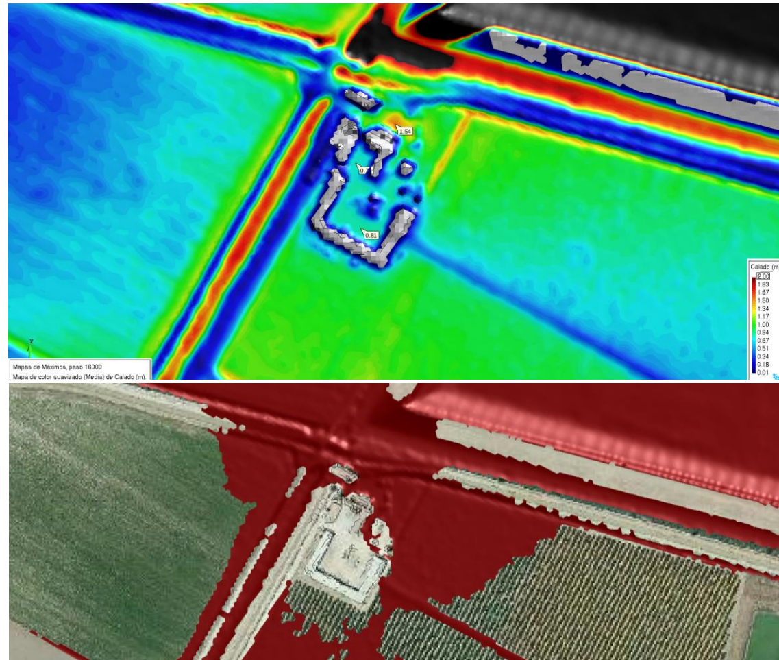
Figura 58. Ampliación de calados máximos Zonas de graves daños en el Cortijo Las Lomas (rotura 3)
