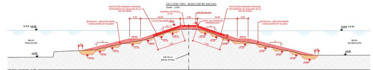
Figura 51. Secciones tipo del recrecimiento del dique entre las balsas de regulación y decantación.
