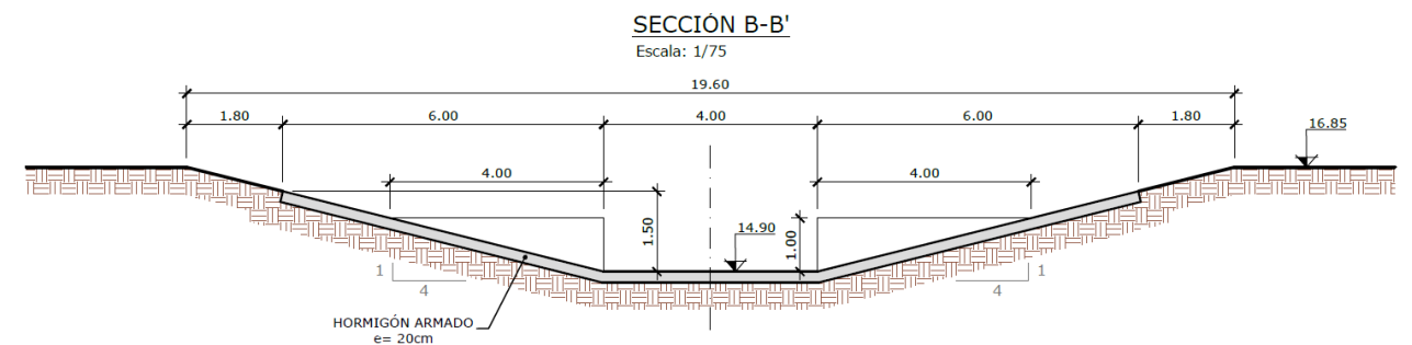
Figura 46: Aliviadero balsa de regulación. Planta. S, Alcantarillas
