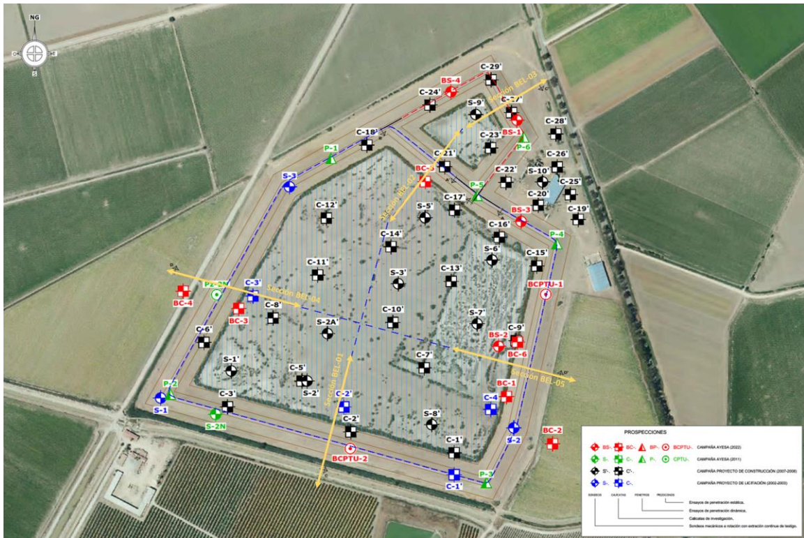
Figura 55. Imagen de la Balsa de Belmonte con indicación de los trabajos realizados y secciones de cálculo.
