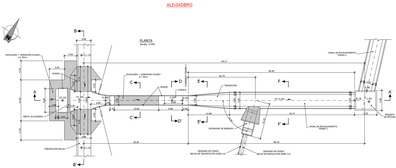
Figura 33: Aliviadero balsa de regulación. Planta. S, Belmonte
