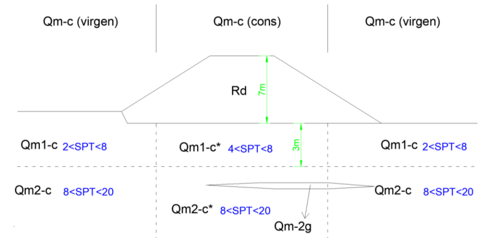
Figura 52. Esquema localización unidades geotécnicas
