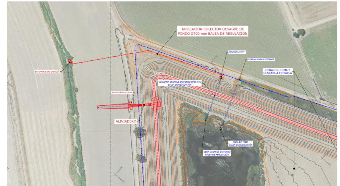
Figura 48: Diseño de la prolongación del desagüe de los nuevos desagües de fondo de la balsa de decantación y regulación
