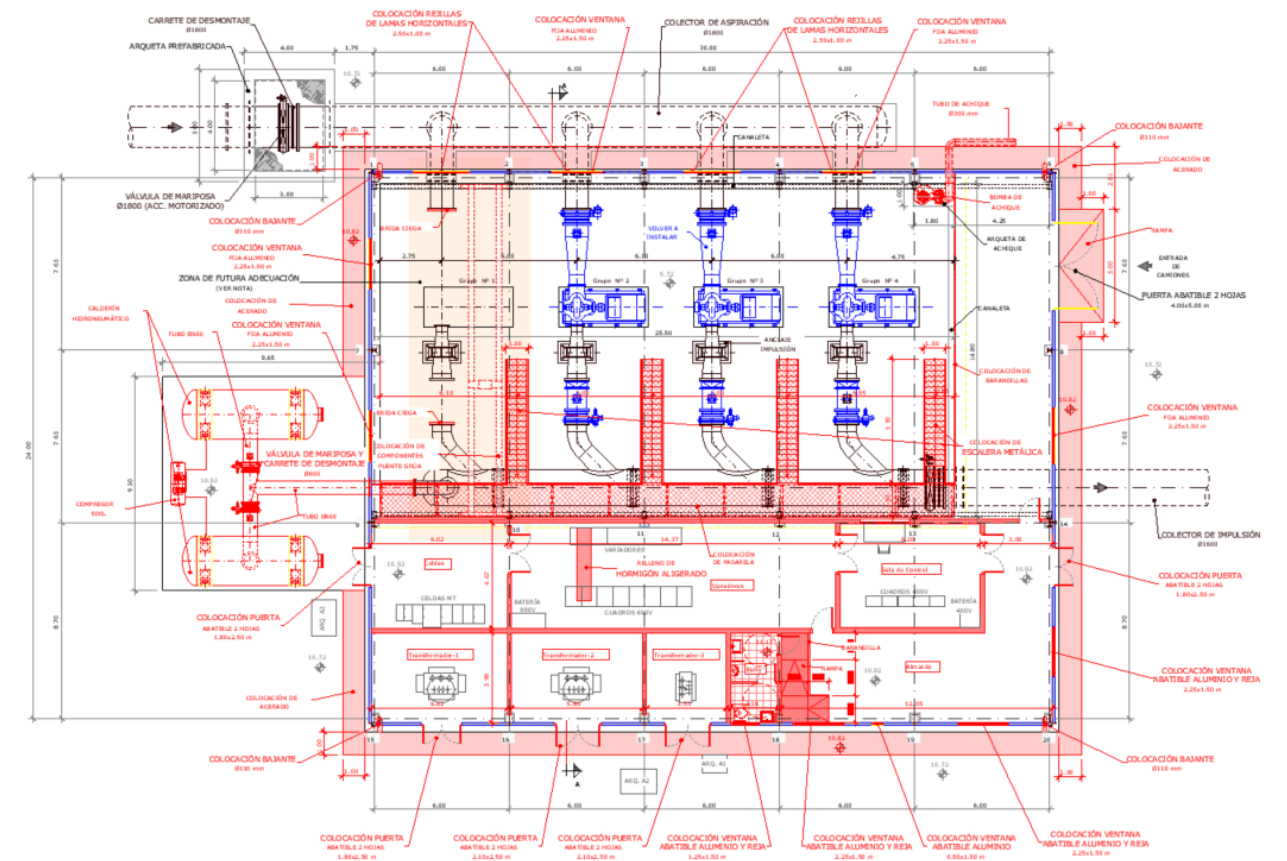
Figura 49. Planta de la estación de bombeo.
