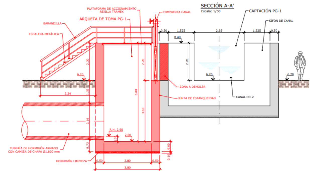
Figura 27. Nueva obra de captación en canal de derivación CD-2 (Pico Gorrión)
