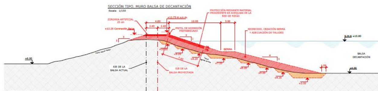
Figura 30. Sección tipo. Dique recrecido de la balsa de decantación
