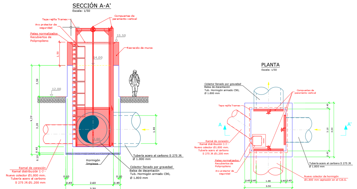
Figura 43; Ramal de conexión by-pass del bombeo, para enviar agua al CBG en gravedad. Ya ejecutado
