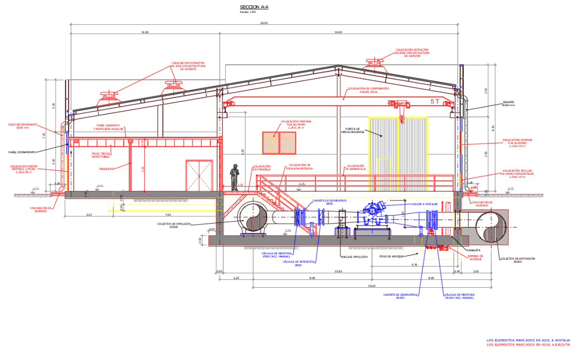
Figura 38. Perfil longitudinal de la estación de bombeo.
