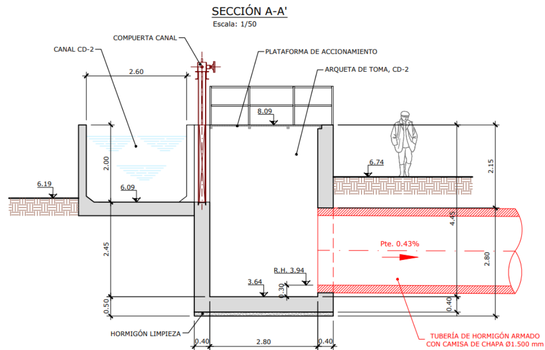
Figura 25. Obra de captación en canal de derivación CD-2. Existente ya ejecutada
