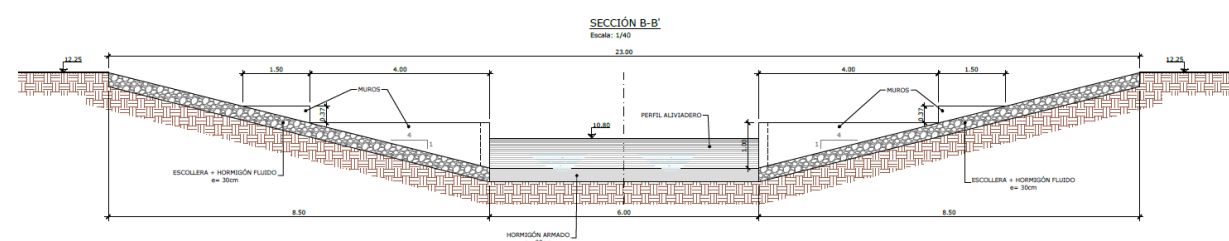
Figura 32: Aliviadero balsa de regulación. Alzado
