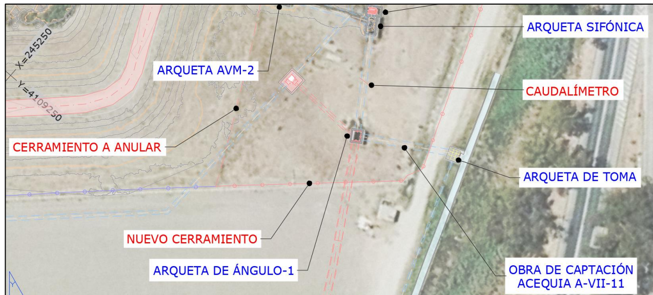
Figura 42; Ramal de conexión by-pass del bombeo, para enviar agua al CBG en gravedad. Nueva obra
