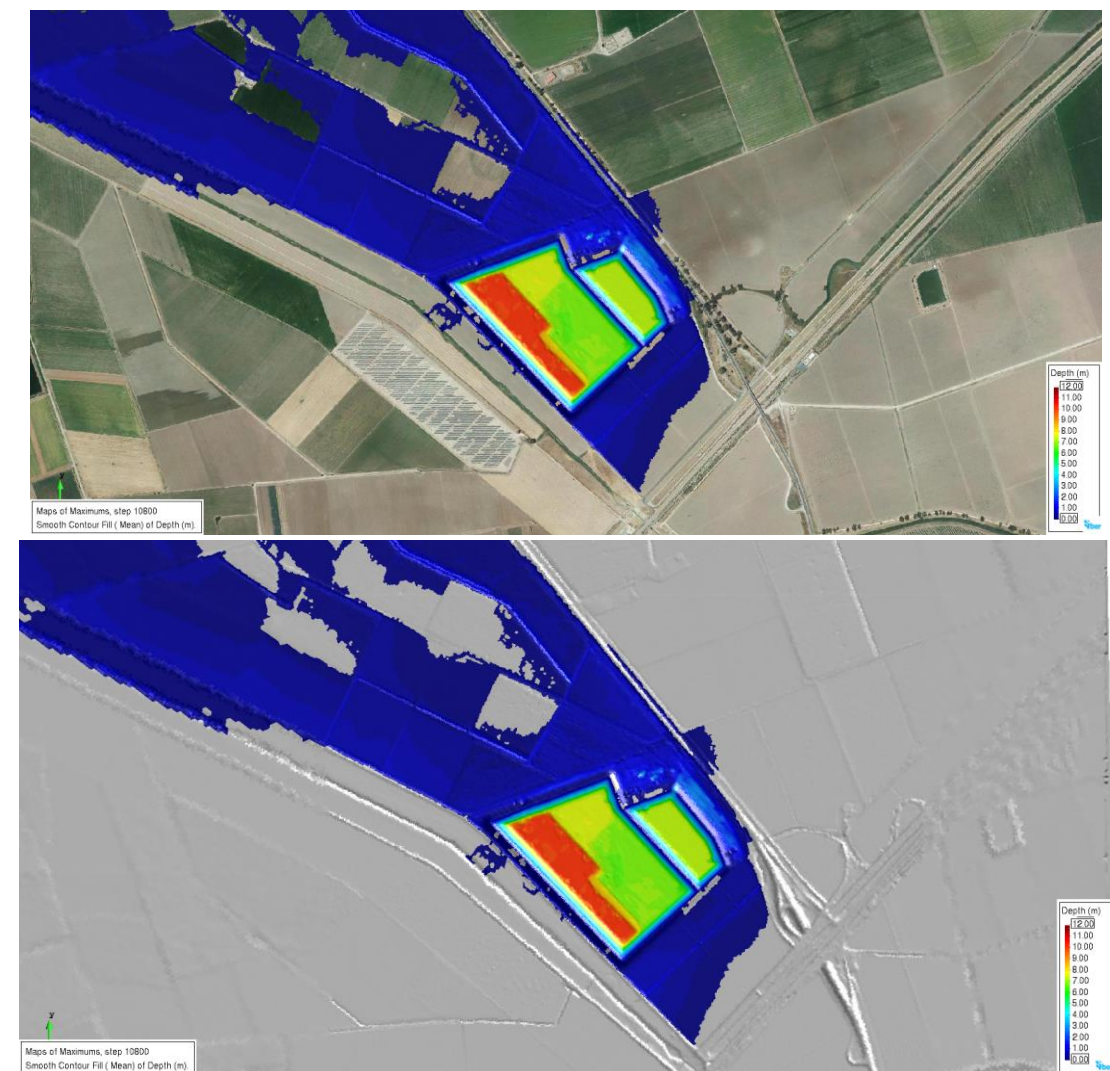
Figura 60. Máximos calados alcanzados en la rotura 4 estado actual
