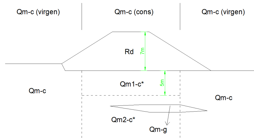
Figura 56. Esquema localización unidades geotécnicas
