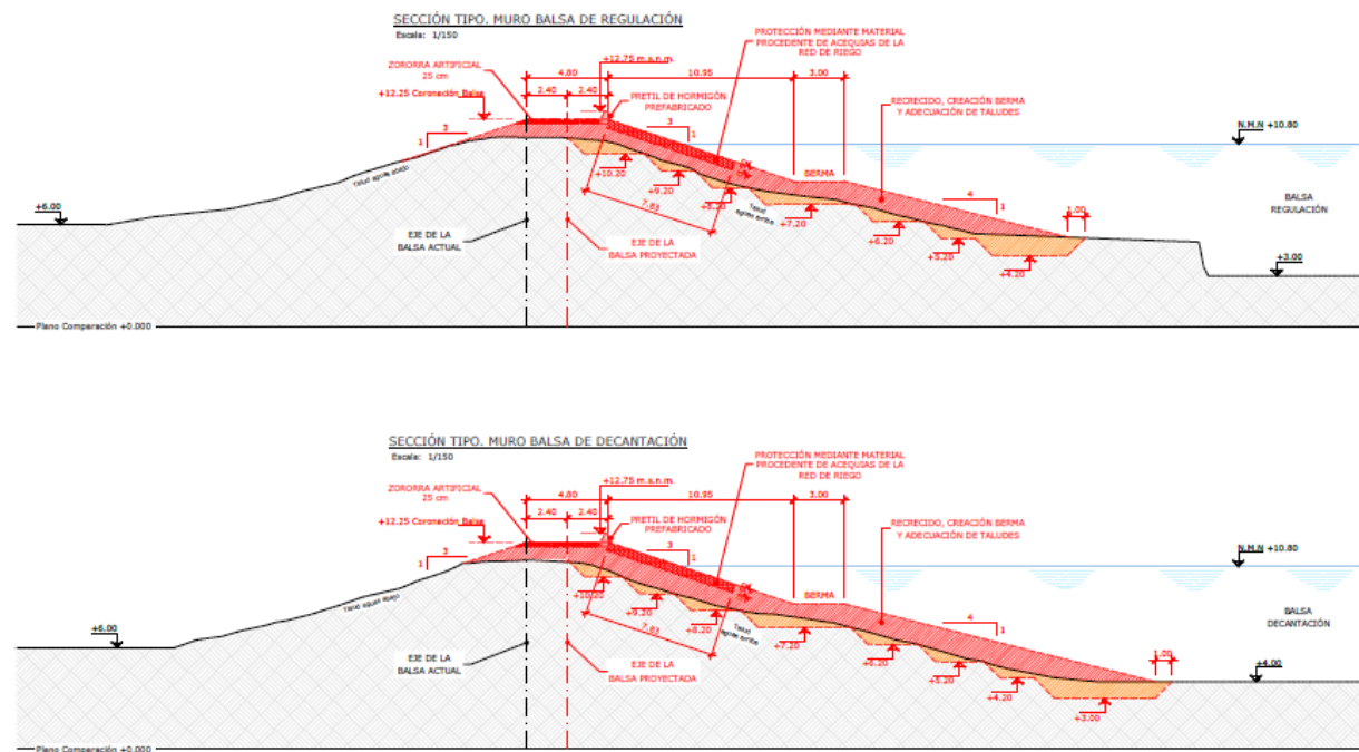
Figura 50. Secciones tipo del recrecimiento de los diques externos de las balsas de regulación y decantación de Belmonte.
