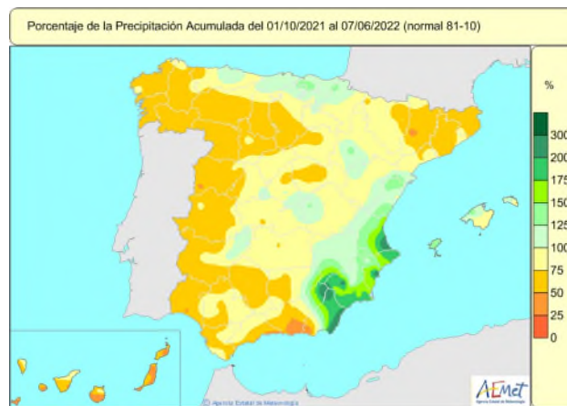
Mapa 4: Hace 2 años
