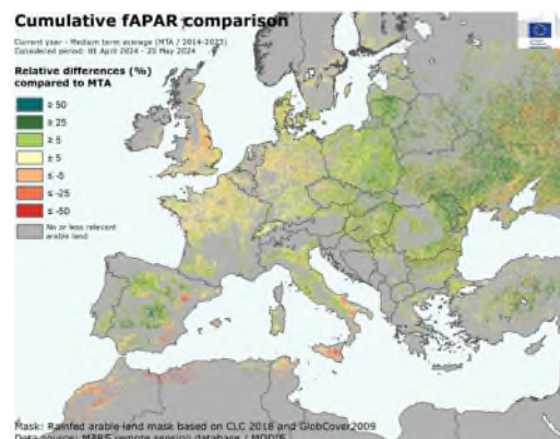
Mapa 3: Índice fAPAR
