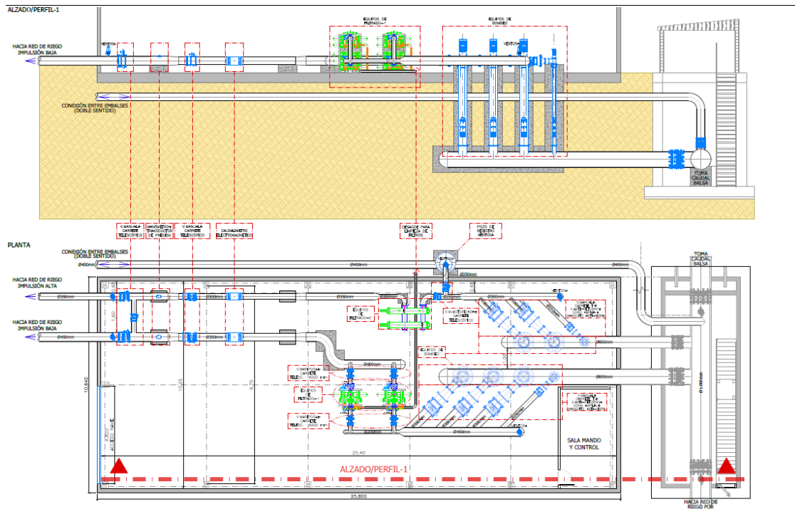
Figura 2: Planta de la distribución de las instalaciones en la nave de bombeo.
