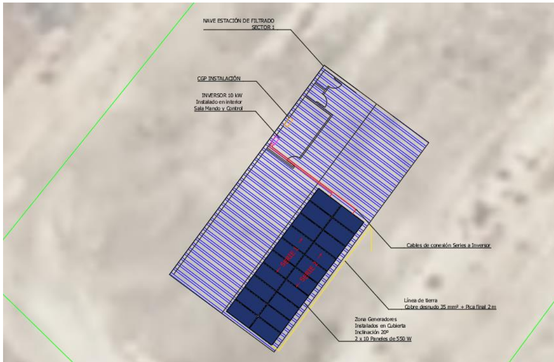
Figura 7: Planta general de la instalación fotovoltaica proyectada para la estación de filtrado
