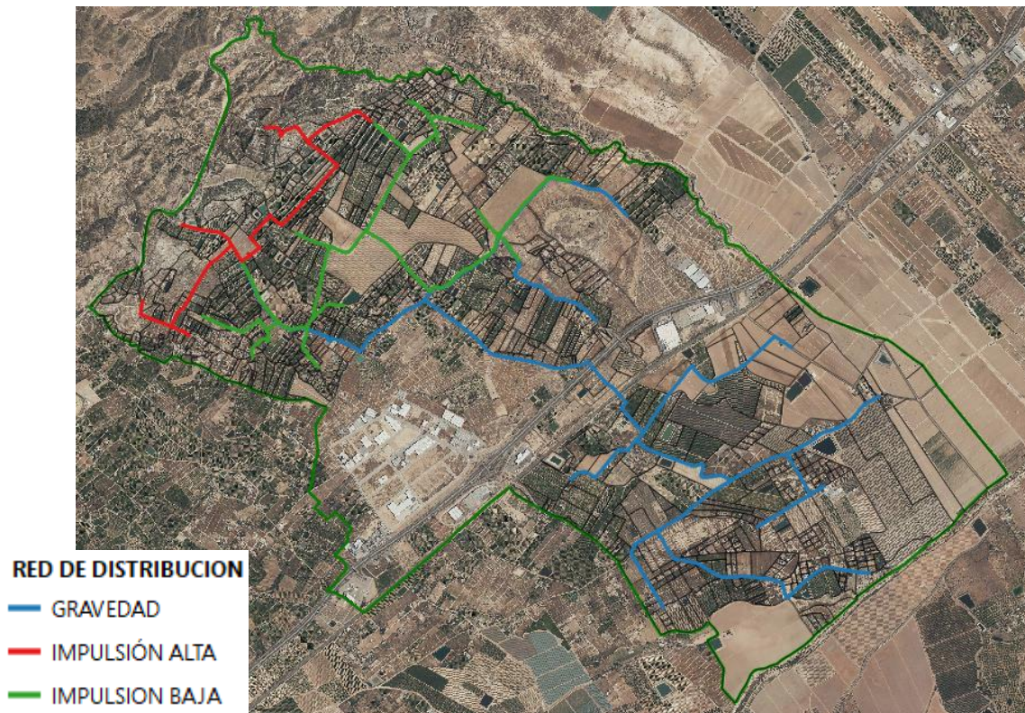
Figura 8: Planta de la red de distribución de las diferentes zonas de riego.
