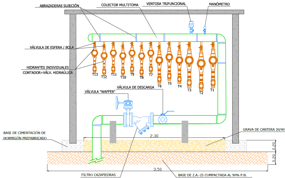
Figura 9: Detalle de las casetas propuestas
