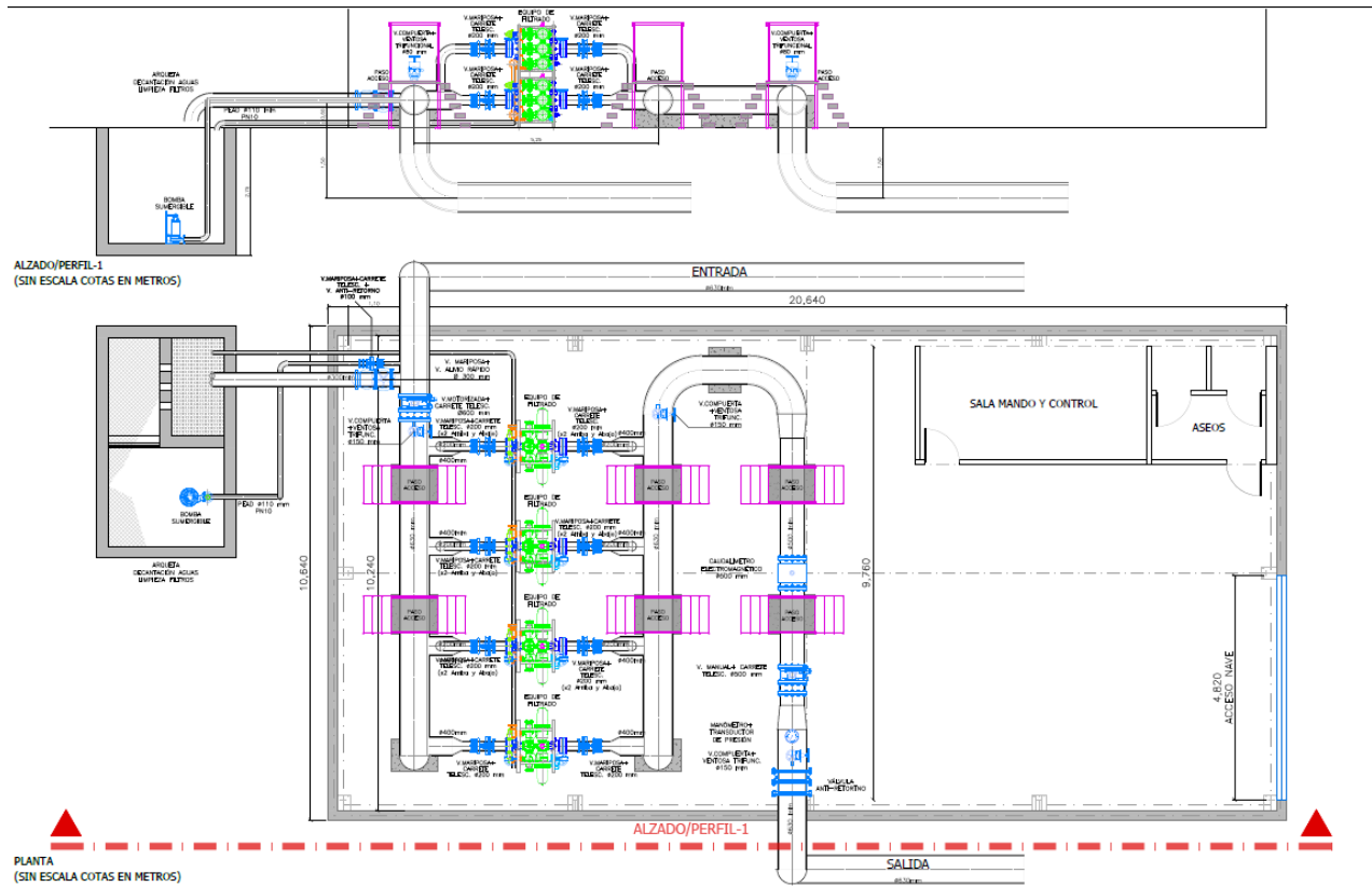
Figura 3: Planta de la distribución de las instalaciones en la nave de gravedad.
