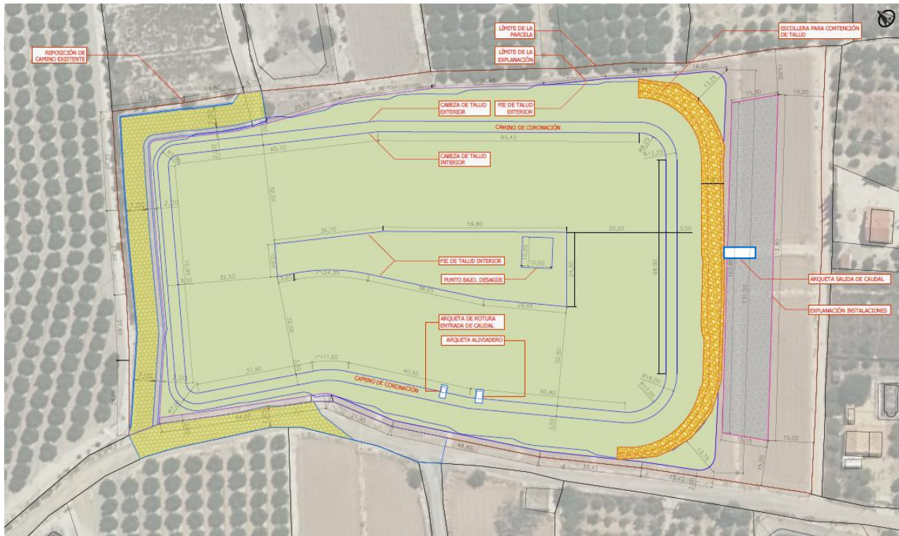
Figura 1: Vista general de la balsa proyectada.
