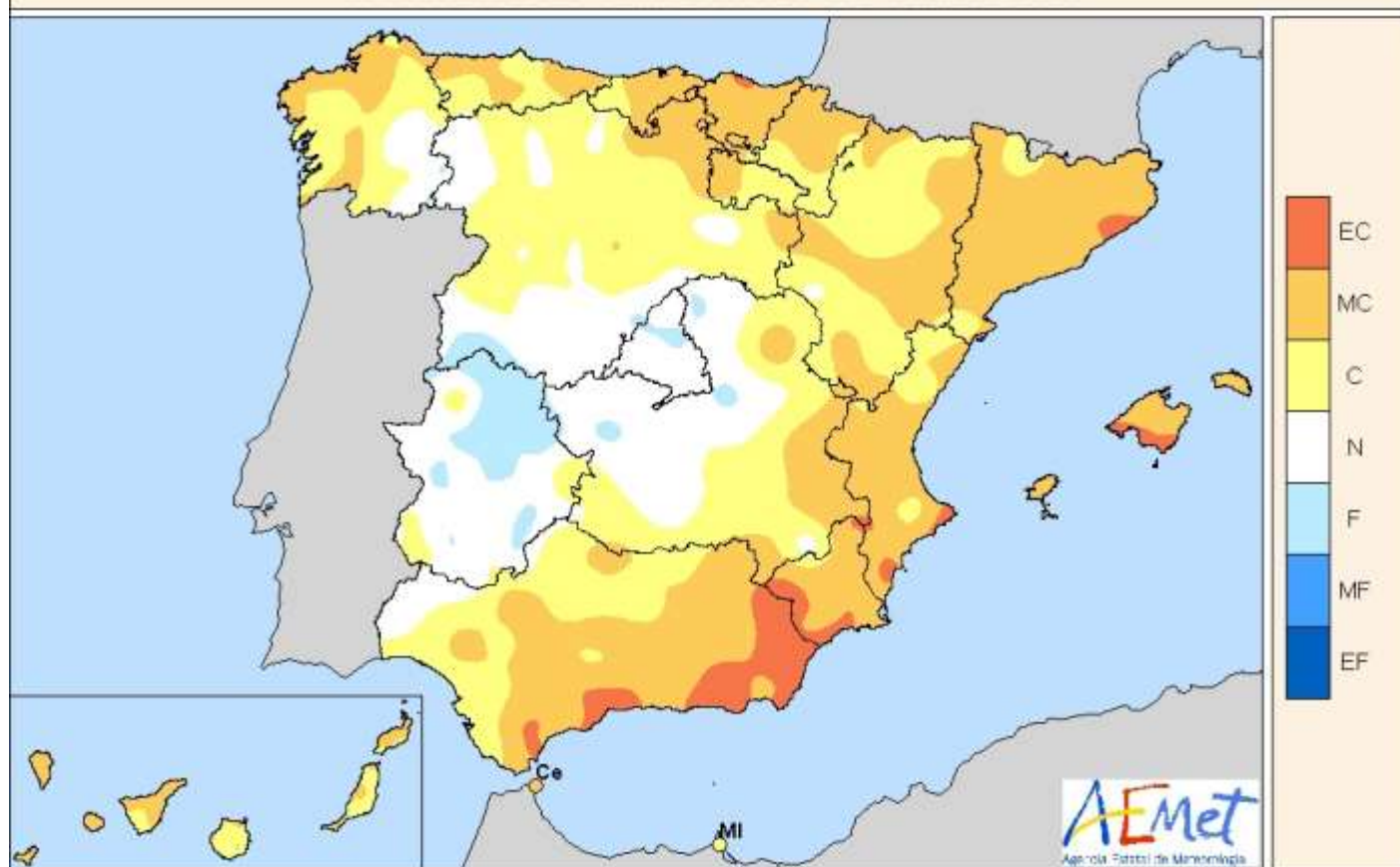
CARÁCTER DE LA TEMPERATURA - SEPTIEMBRE 2021
