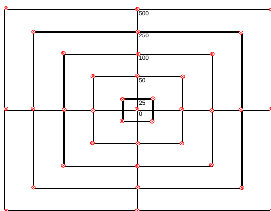
Figura 1: Red de trapeo para A. ludens , distancia en metros. Superficie total, 1 Km 2 .
