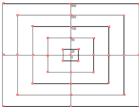
Figura 2: red de trampeo (Zona infestada) para A. ludens , distancia en metros. Superficie total, 1 Km².
